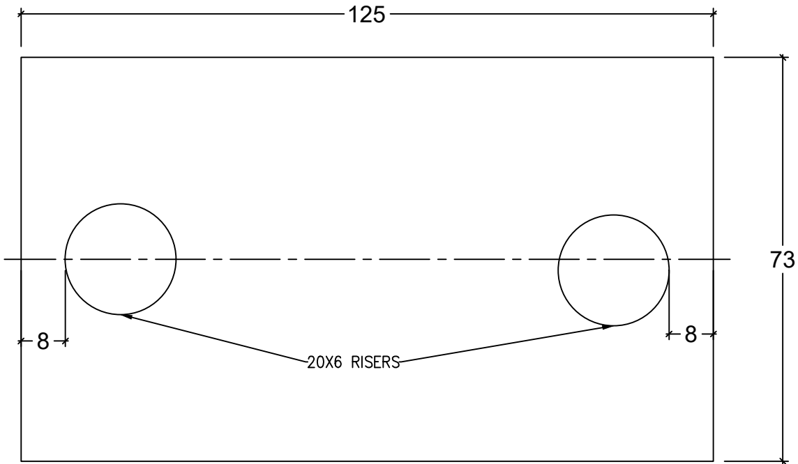
LID TOP VIEW
